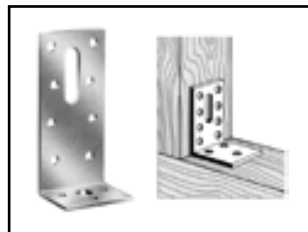
Ъглова връзка (винкел) - несиметрична
