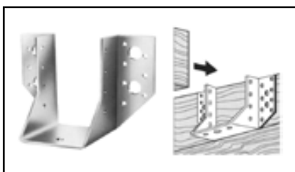
Обувка за греда, тип А
