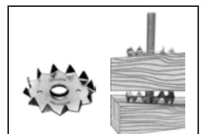
Връзка - булдогов едностранен и двустранен
